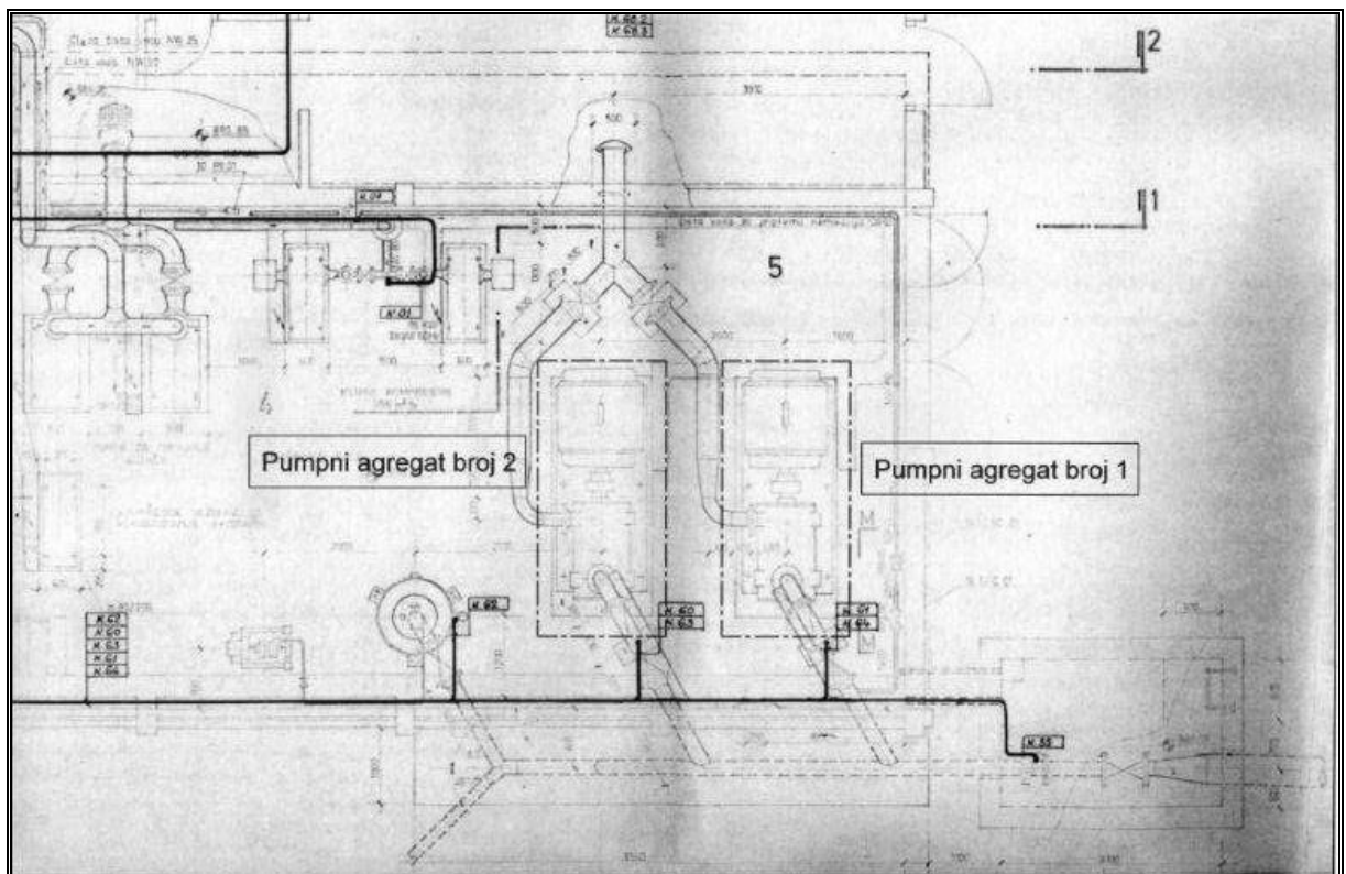
Слика број 1 - Пумпна станица чисте воде
