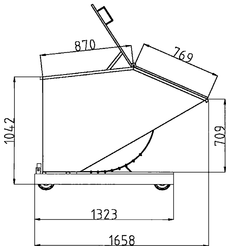
Нагибни кип контејнер са поклопцем 1м 3 – поглед 1
