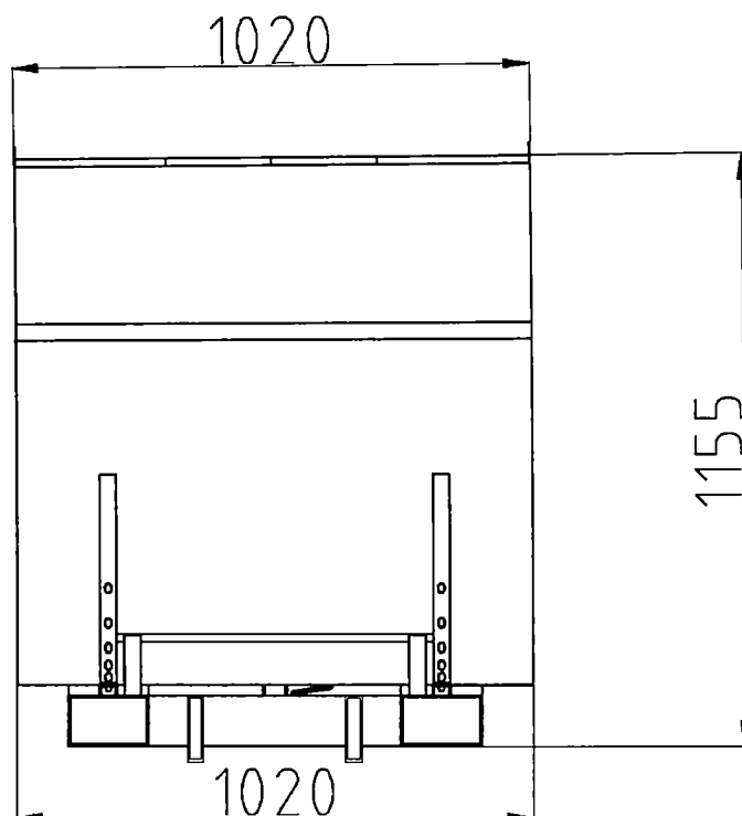
Нагибни кип контејнер са поклопцем 1м 3 – поглед 2
